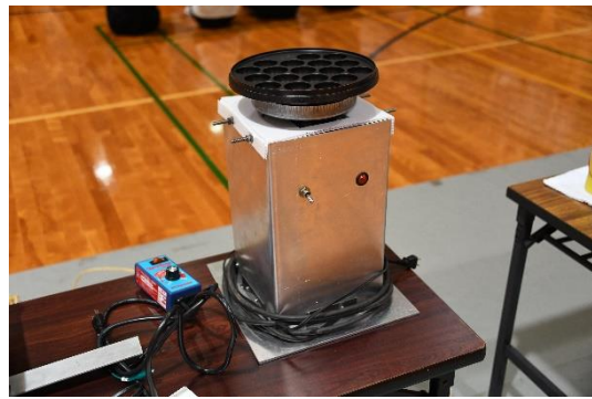
自動たこ焼き器
