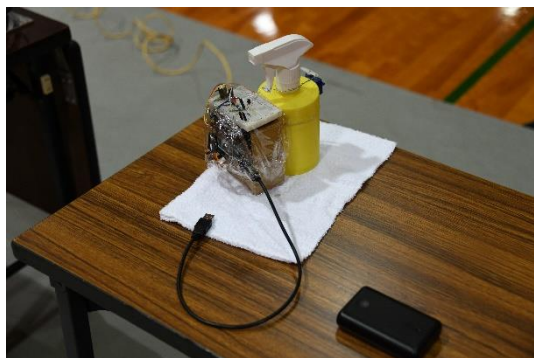
自動アルコール噴射機
